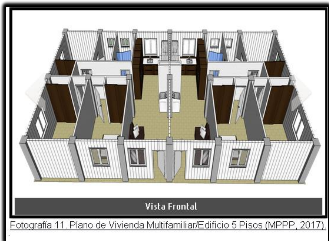
Fotografía 11. Plano de Vivienda Multifamiliar/Edificio 5 Pisos (MPPP, 2017).
