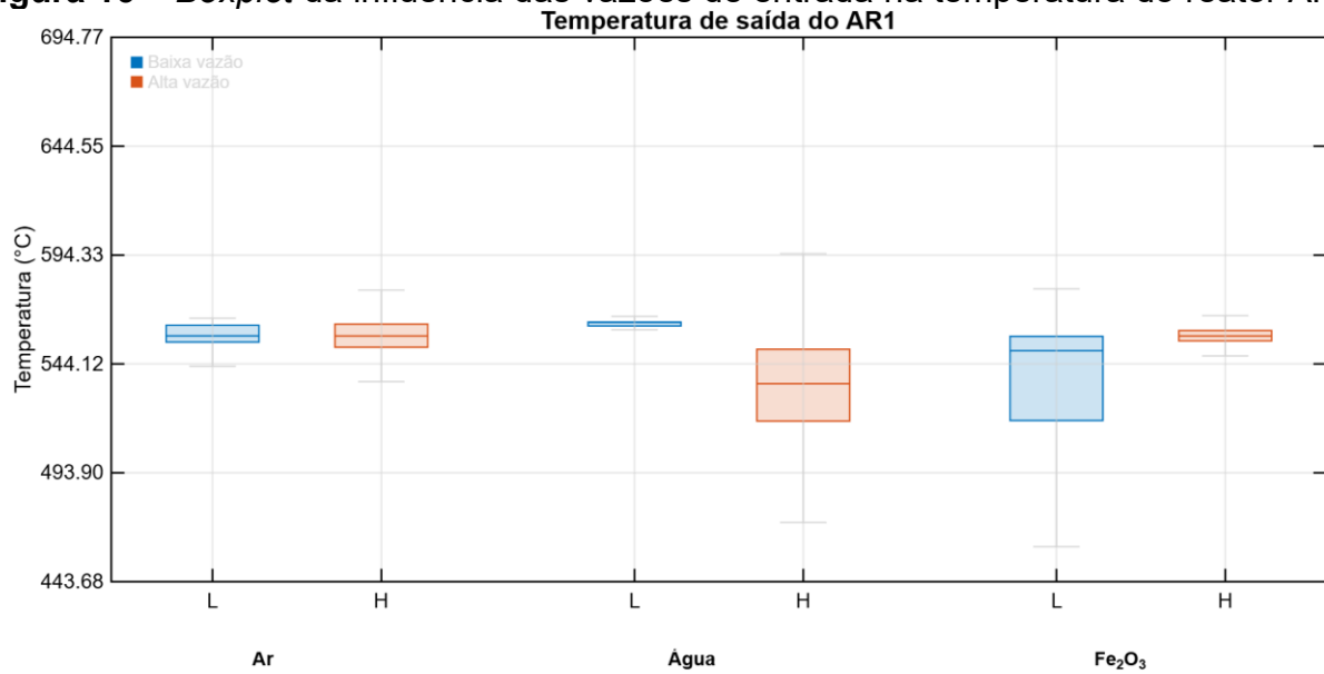
Figura 16 – Boxplot da influência das vazões de entrada na temperatura do reator AR1.
