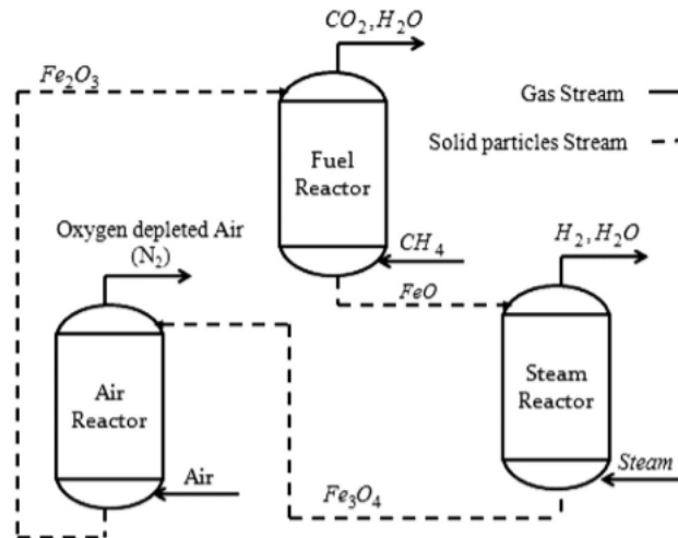
Figura 3 – Configuração de TRCL utilizando um OC a base de ferro
