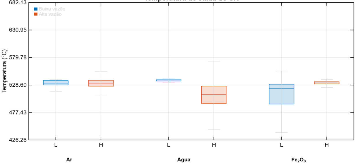
Figura 15 – Boxplot da influência das vazões de entrada na temperatura do reator SR. Temperatura de saída do SR
