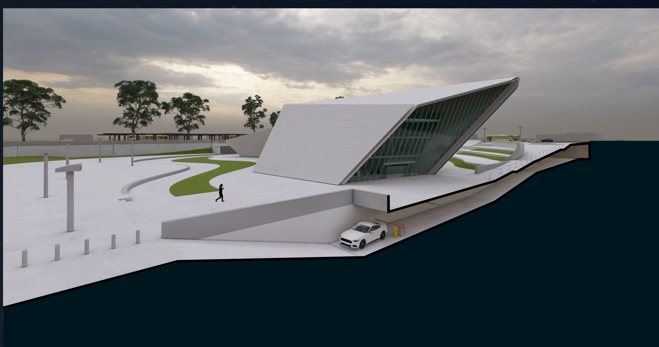
CORTE A-A (ACESSO VEÍCULOS)
