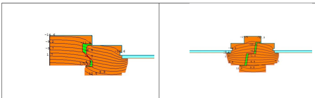
Figura 1a. Planta: Cálculo para o batente esquerdo para a caixilharia em madeira e vidro.
