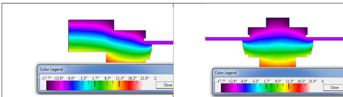
Figura 1a. Planta: Cálculo para o batente esquerdo para a caixilharia em madeira e vidro.
